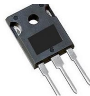
IRFP450 MOSFET N 14A 500V 190W 0.4E
