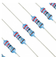
RE391F RESISTENCIA METALFILM 0.4W 1% 390 OHM
