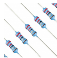
RE122F RESISTENCIA METALFILM 0.4W 1% 1K2
