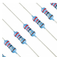
RE474F RESISTENCIA METALFILM 0.4W 1% 470K
