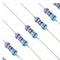
REPI-12K RESISTENCIA METALFILM 1W 5% 12K
