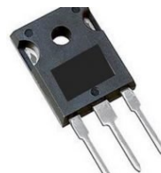
IRFP150 MOSFET N 40A 100V 0.055E TO-3P
